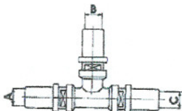
4031 Raccordo tee maschio. Male tee fitting.
